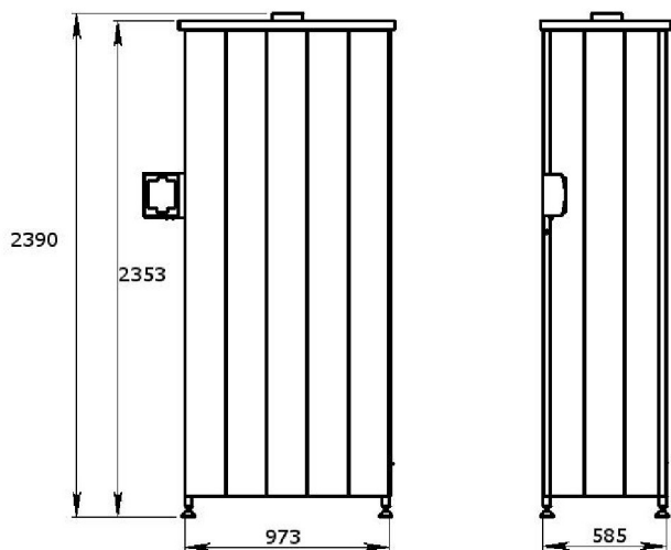
Code 18769 Armoire 24 paires
