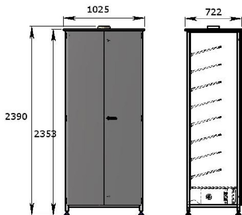
Code 18908 Armoire 24 paires
