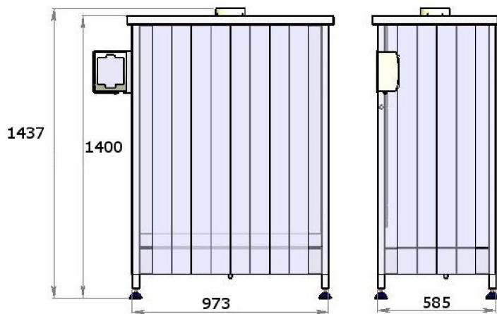
Code 18759 Armoire 12 paires
