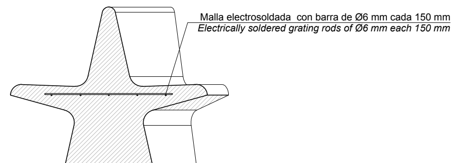
SECCIÓN / SECTION
