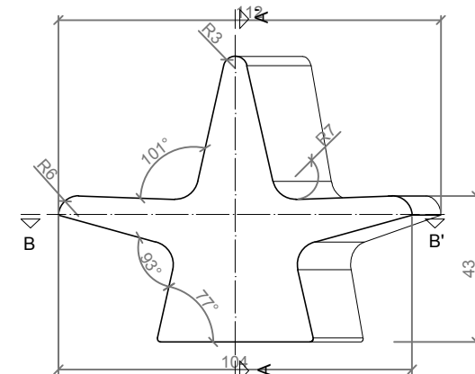
PERFIL / RIGHT SIDE
