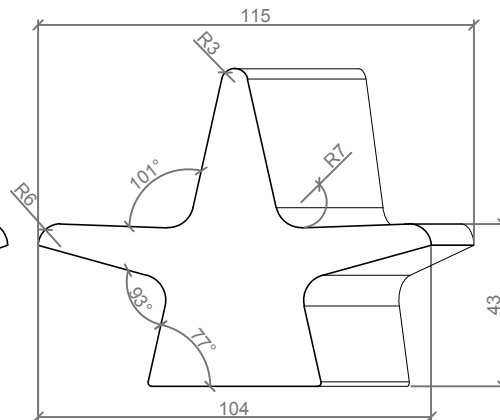
PERFIL / RIGHT SIDE
