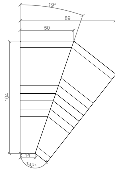
PLANTA / TOP VIEW
