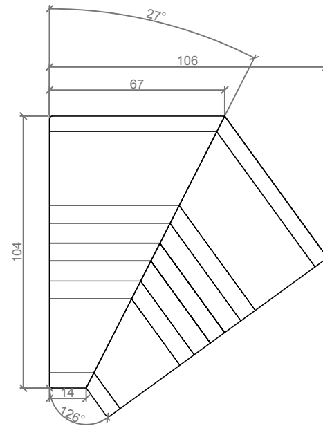
PLANTA / TOP VIEW
