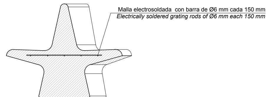
SECCIÓN / SECTION
