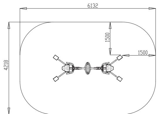
Zone de sécurité - Echelle 1:100
