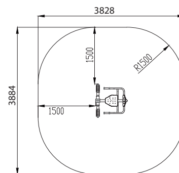
Zone de sécurité - Echelle 1:100
