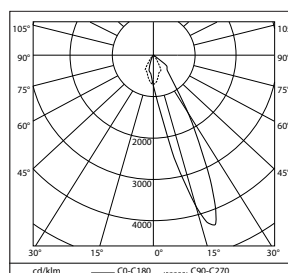
Diffusion lumineuse LED 5,4 W.
