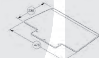
Bavette GS-NG 476 x 239 x 7 mm, pour les produits conditionnés en cartons (par ex. boîtes de boissons), référence 930 084
