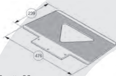
Bavette GS 476 x 239 x 7 mm, utilisée entre autre dans l'industrie des boissons. Suffisamment large pour assurer la stabilité des fûts et des caisses lors de la manutention, référence 930 030
