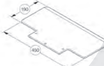
Bavette DS-NG 450 x 190 x 7 mm, également pour les produits conditionnés en cartons, référence 930 085
