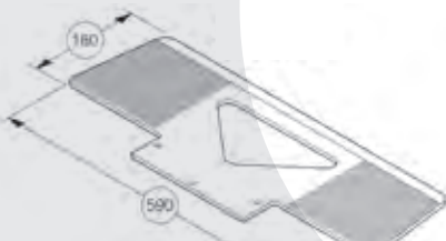
Bavette XWL 590 x 180 x 7 mm, également pour les produits blancs, avec pieds sur bavette! référence 930 074
