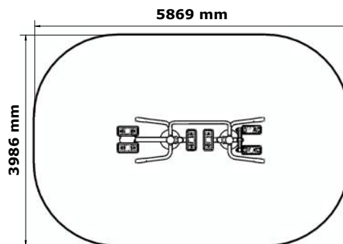
Zone de sécurité - Echelle 1:100
