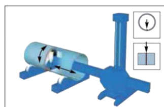
Soudure interne - axiale et circulaire
