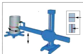
Soudure circulaire et verticale vers le bas, sur la table tournante
