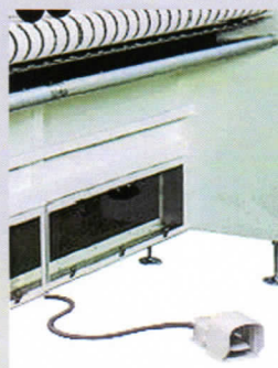
Barre de roulettes d'engagement avec roulettes indépendantes sur toute la largeur de la voie, conseillée pour les tabliers et nappes.
