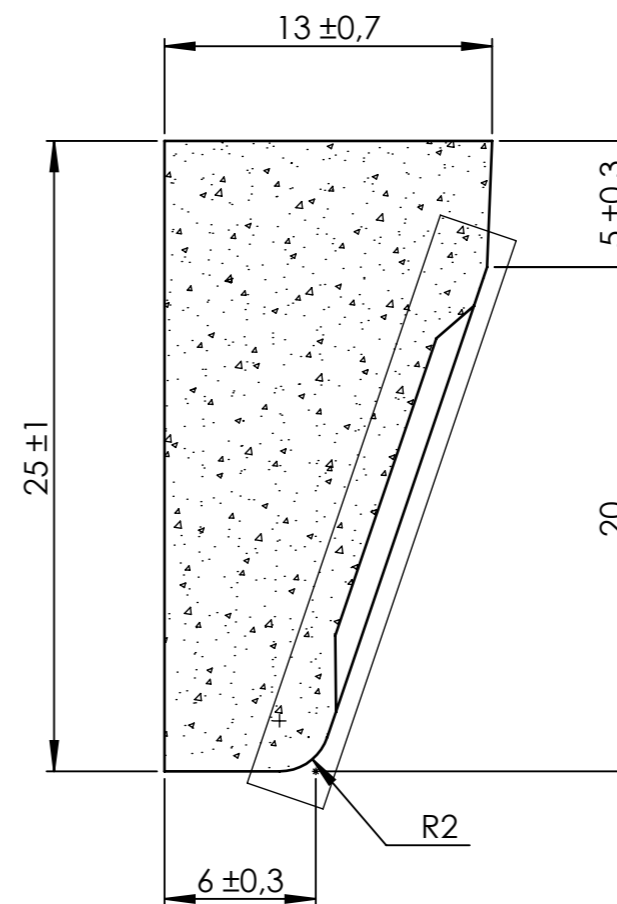
COUPE A-A
