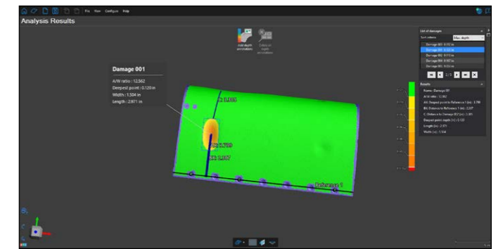
Enfoncements sur le bord d'attaque d'une aile d'avion mesurés avec le module Aerospace de VXintegrity
