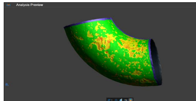
Corrosion sur un sol de réservoir analysée avec le module Damage Monitoring de VXintegrity
