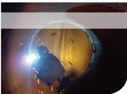
[ Pose d'une cloison acier ]
