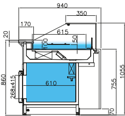
LCVT - VUV 3M2 ventilada total total ventilated ventilée totale ventilada total
