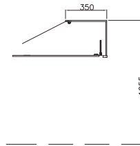
OPÇÃO: VDB vidro direito baixo desmontável demountable low flat front glass vitrage droit bas amovible vidrio reto bajo desmontable
