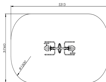
Zone de sécurité - Echelle 1:100
