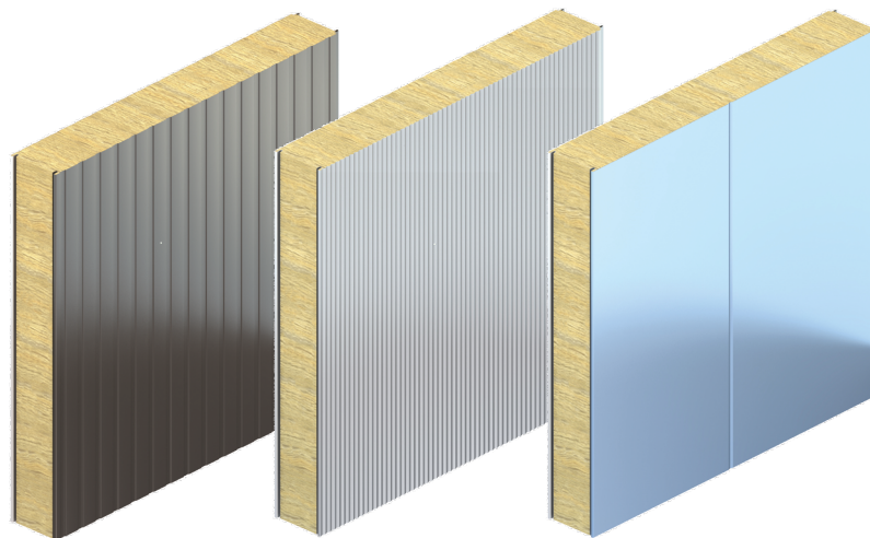
Profil nervuré
