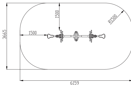
Zone de sécurité - Echelle 1:100
