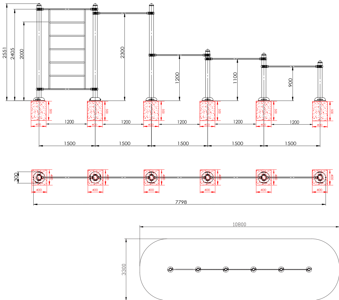
Zone de sécurité - Echelle 1:100
