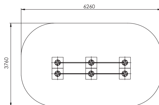
Zone de sécurité - Echelle 1:100
