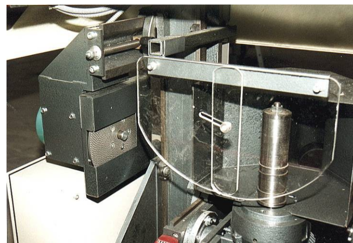
Vue de détail d'une épaveuse à l'arrière avec disque à plaquettes carbure (option)
