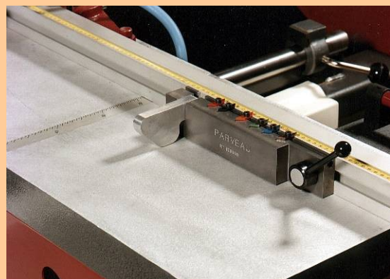
Règle aluminium inclinable de 0 à 50° avec butée escamotable et repères de coulures
