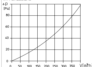
Druckverlust Außenluft-Ansaugsäule mit Filter G3* und 40 Meter Erdkollertorrohr im Reinzustand
