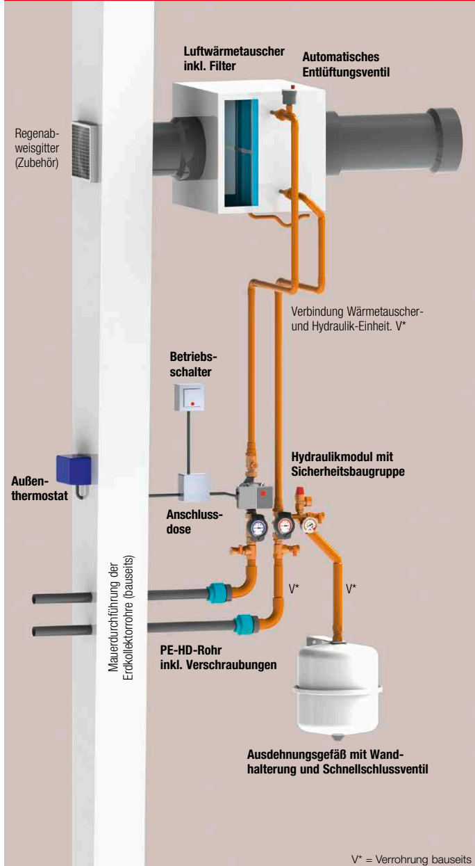
SEWT-Bausatz Best.-Nr. 02564
