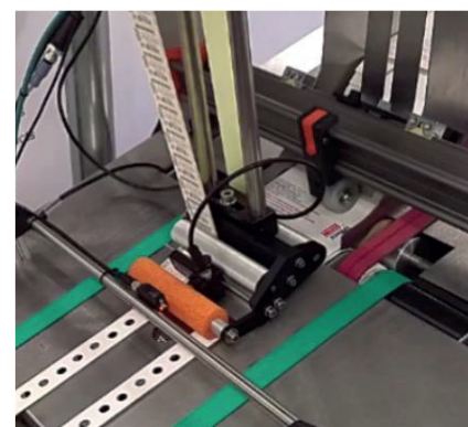
Module d'étiquetage
